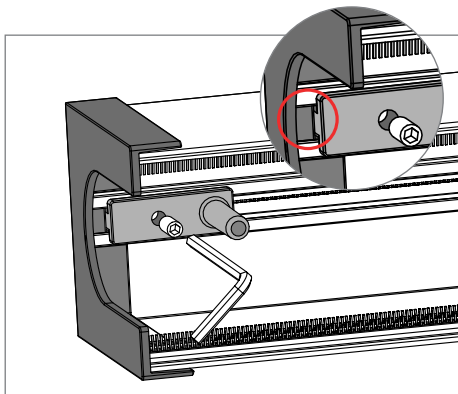
5 Posizionare la baionetta in battuta con il tappo (il dentino - in rosso - funge da dima) e solo dopo fissare con il grano.
