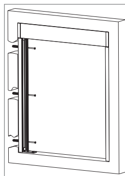
9 Fissare il profilo laterale, praticando dei fori.
