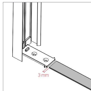
12 Rimuovere la pellicola protettiva del biadesivo dalla guida inferiore, applicare a pavimento la guida tra i due profili laterali. Applicare la guida in battuta lasciando un margine di 3 mm dall'aggancio inferiore.
