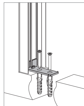
10 Fissare l'aggancio al vano.
