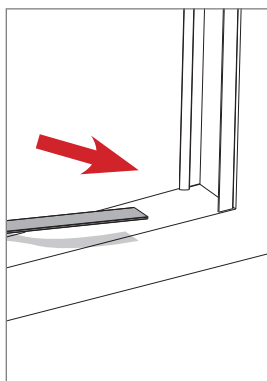
12 Rimuovere la pellicola protettiva del biadesivo dalla guida inferiore, applicare a pavimento la guida tra i due profili laterali. Applicare la guida in battuta lasciando un margine di 3 mm dall'aggancio inferiore.
