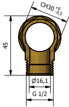
A-A ( 1 : 1.5 )
