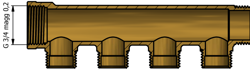
B-B ( 1 : 1.5 )
