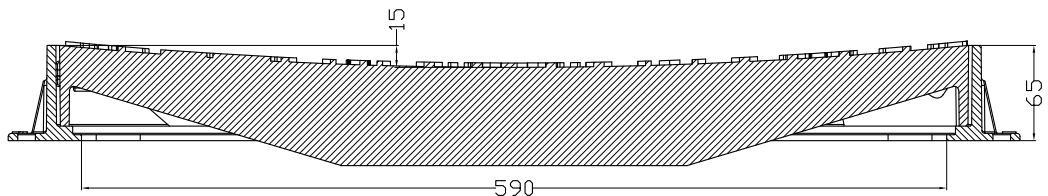
SEZIONE A-A
