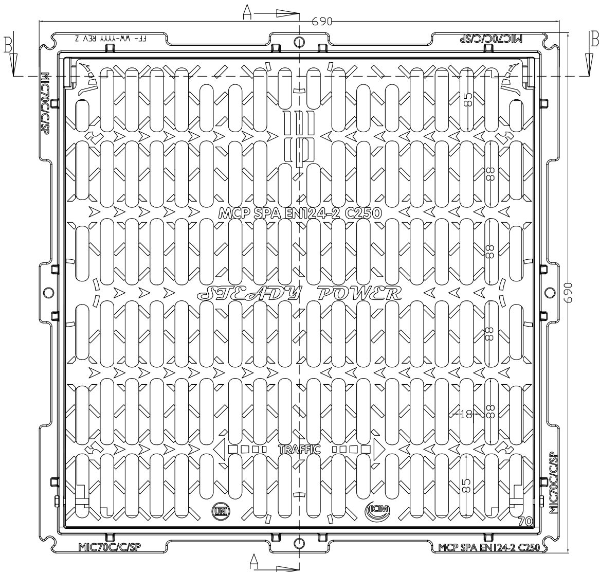
VISTA SUPERIORE
