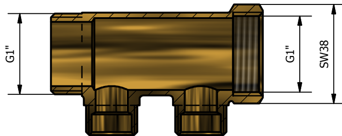
B-B ( 1 : 1.5 )
