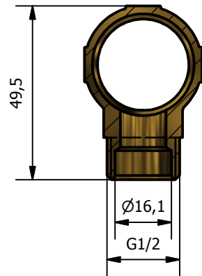
B-B ( 1 : 1.5 )
